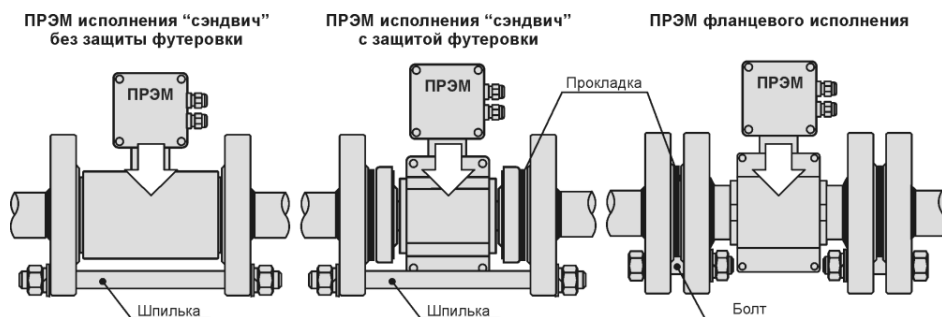
Рисунок 2 – Варианты монтажа ПРЭМ
