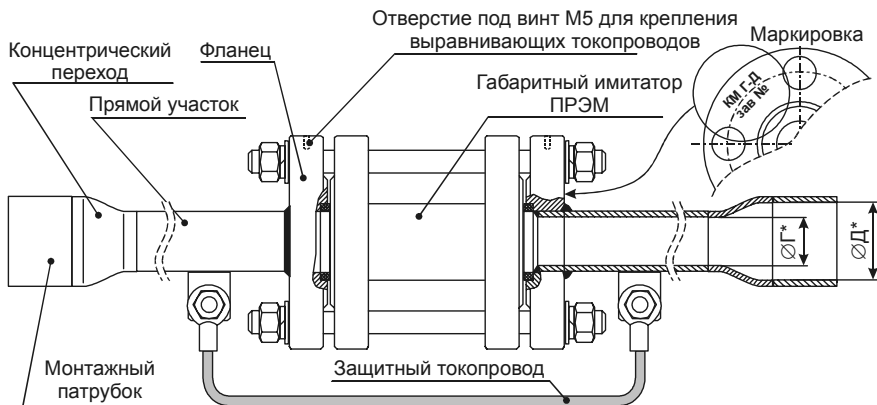
Рисунок 1 – Внешний вид КМ
